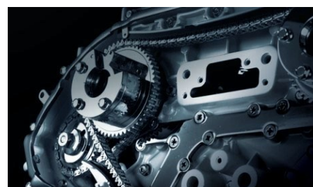
Новый бензиновый двигатель 1.6 H4M 113 л.с. с цепным приводом ГРМ
